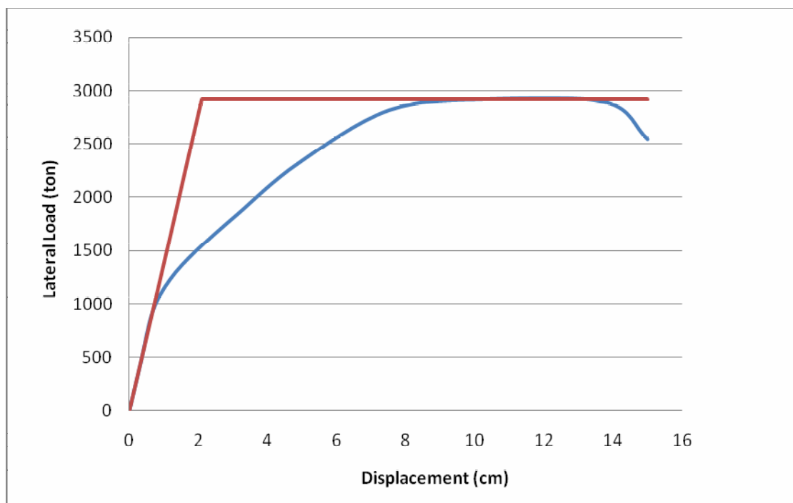
شکل خ-۲۸- منحنی تغییرات بار جانبی کل (برش پایه) برحسب تغییرمکان و داشته برای مجموعه پایه‌های پل
