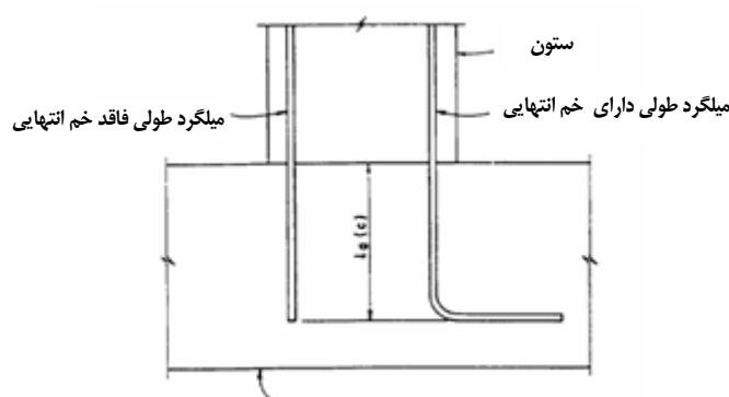
شالوده (در انتهای تحتانی) یا سر ستون (در انتهای فوقانی) شکل ت-۱۵- طول مهار مؤثر آرماتور طولی در فونداسیون
