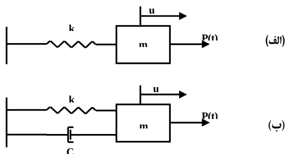
شکل الف-۱-الف): سیستم جرم و فنر، (ب): سیستم متشکل از جرم، فنر و میراگر لزج
