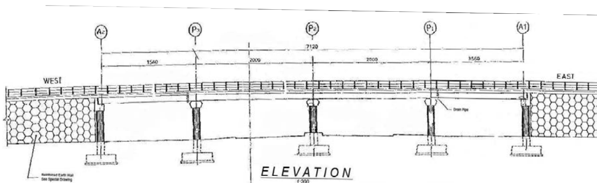
شکل خ-۱- نمای جانبی پل [۵]
