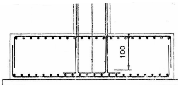
شکل خ-۱۵- طول مهار مؤثر آرماتورهای طولی در شالوده (تنگ ستون‌ها نشان داده نشده‌است) (به‌طوریکه مشاهده می‌شود در تمام عرض شالوده خاموت‌های میانی پیش‌بینی نگردیده‌اند). (همچنین، آرماتور طولی در گونه‌های طرفین پل منظور نشده‌است)
