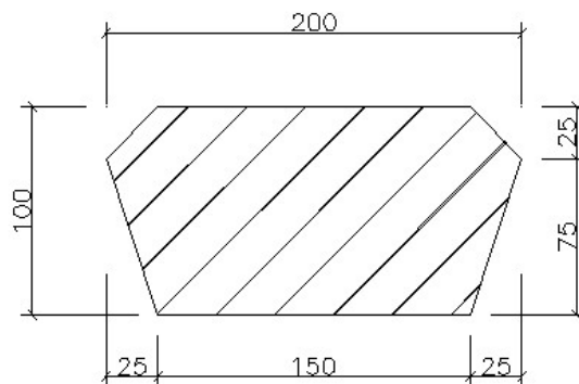
شکل خ-۶- برش سرستون (ابعاد بر حسب سانتی‌متر) [۵]
