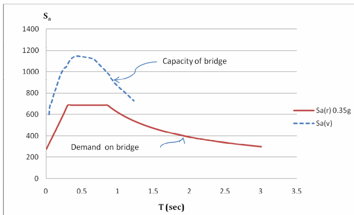
شکل خ-۲۹- منحنی‌های ظرفیت و تقاضای طیفی
