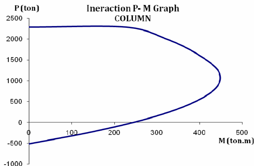
شکل خ-۱۳- منحنی اندرکنش نیروی محوری و لنگر خمشی ستون نمونه (بدون اعمال ضریب کاهش ظرفیت، \phi )
