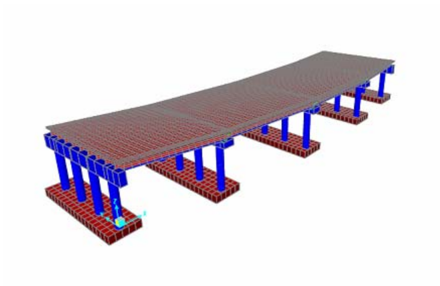
شکل خ-۸- نمای سه بعدی مدل عمومی پل
