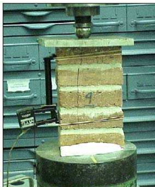
شکل ت-۱-۲ آزمایش تنش فشاری مصالح بر روی نمونه
