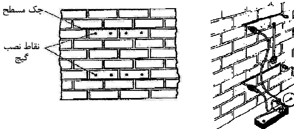
شکل ت-۲-۴ نحوه نصب جک و گيج
