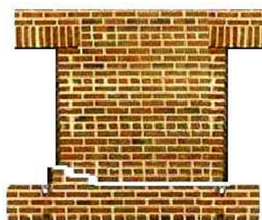
شکل ۱-۴-۲: ترک عمودی در دیوار
