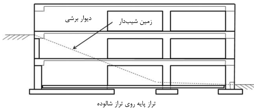
شکل پ ۱-۶ ساختمان با دیوار برشی که فشار جانبی خاک را نیز تحمل می‌کند
