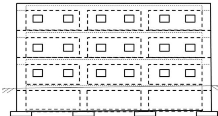
شکل پ ۴-۱ ساختمان با دیوار حایل سرتاسری ناپیوسته با سیستم سازه‌ای
