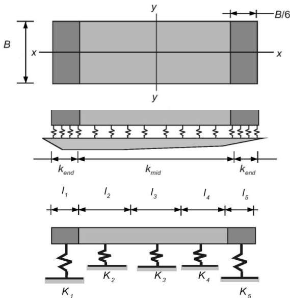
شکل ۲-۵ نمایش فنرهای قائم برای شالوده‌های سطحی صلب
