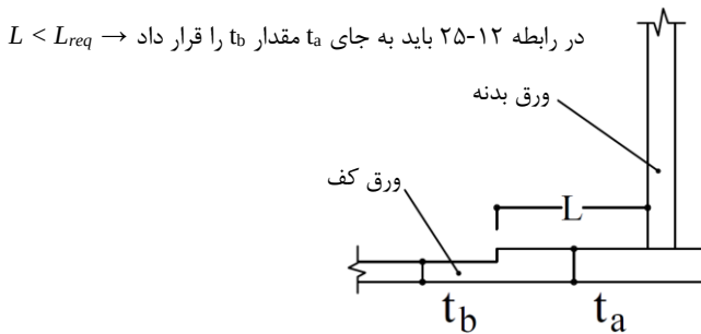
شکل ۲-۱۲ ابعاد ورق‌های بدنه و کف مخزن
