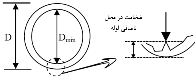
شکل ۱۳-۱ تعیین مقدار D_{min}
