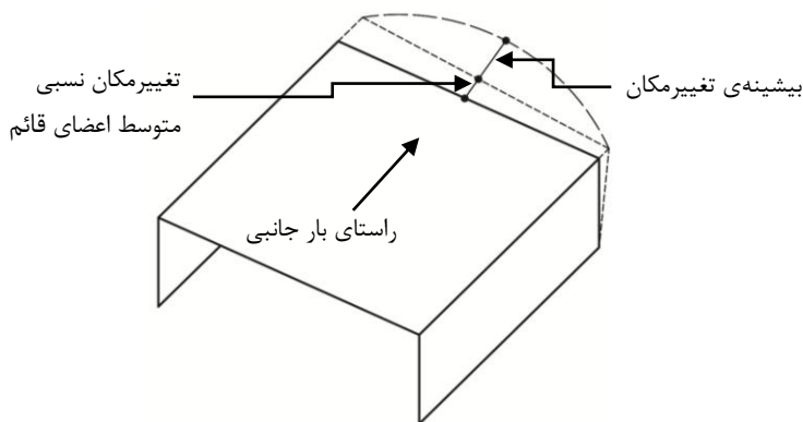
شکل ۳-۴ بررسی صلبیت دیافراگم
