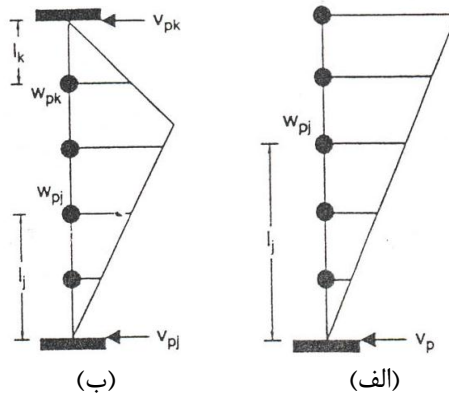
شکل ۸-۱ نمایش شکل مود اول فرضی اجزای غیرسازه‌ای با اتصال در یک یا دو نقطه
