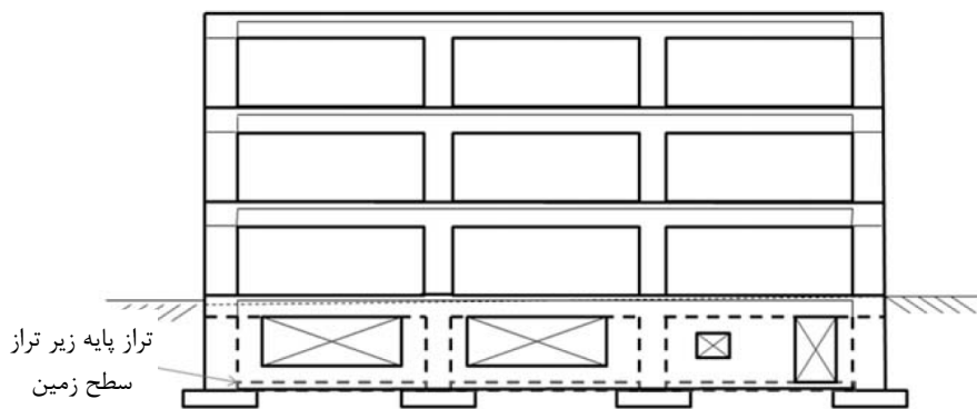
شکل پ ۳-۱ ساختمان دارای باز شو در دیوار حایل
