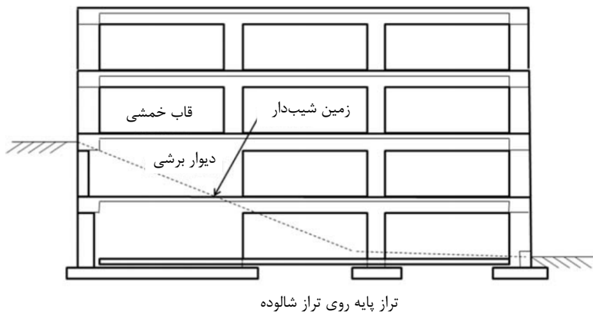
شکل پ ۱-۷ ساختمان با دیوار حایل پیوسته با سیستم سازه‌ای
